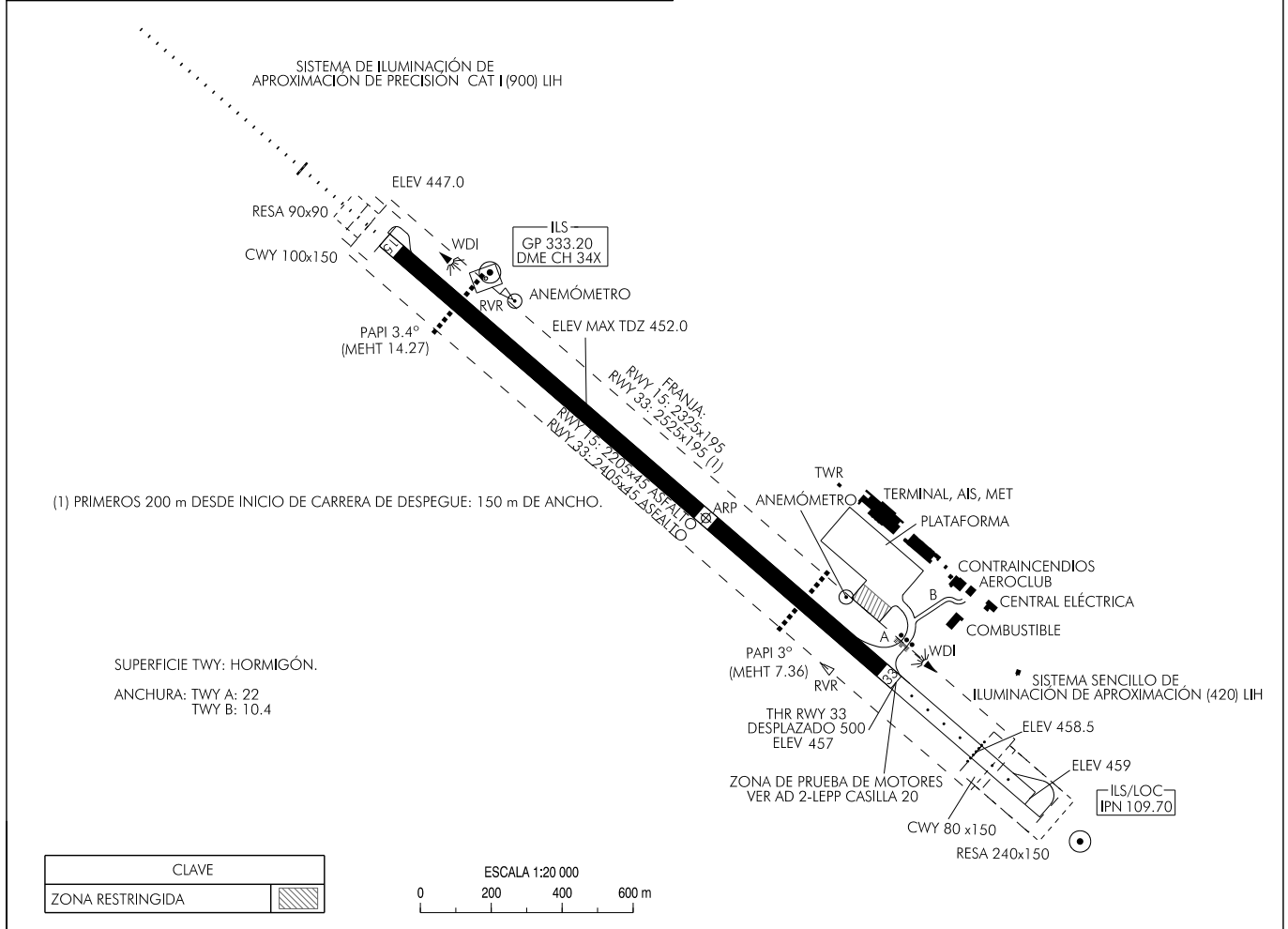
SEÑALES RWY & TWY
